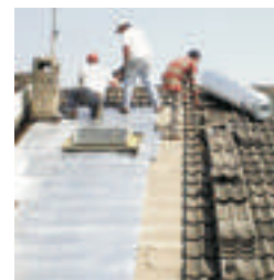
Aplicación Fonpex-ALU+
